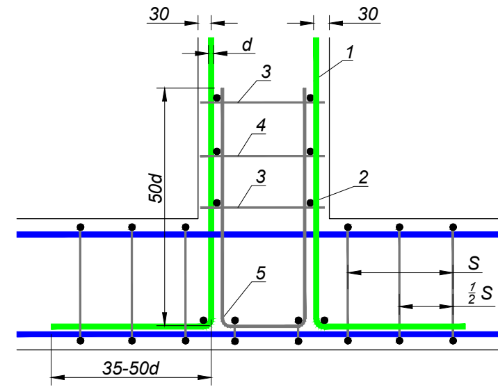
Варіант Д. Армування примикання за допомогою П-подібних хомутів
