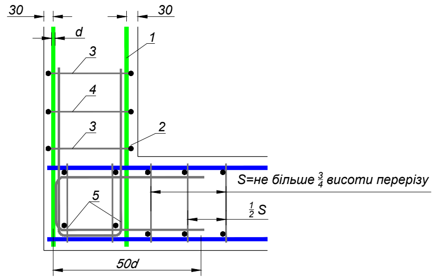
Варіант Г. Армування кута за допомогою П-подібних хомутів
