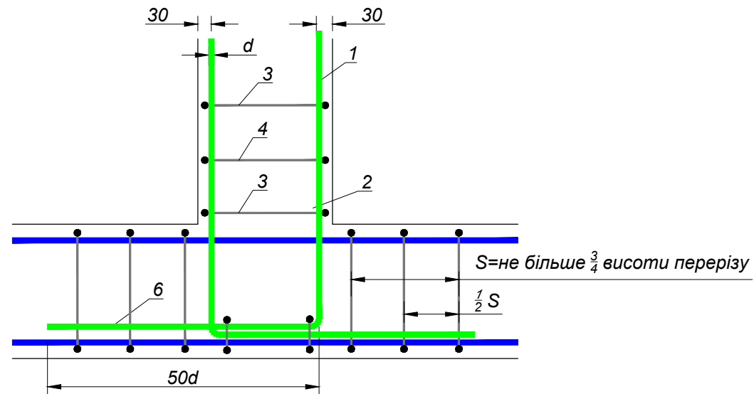
Варіант Е. Армування примикання внапуск
