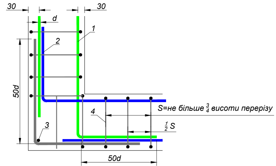
Варіант Б. Армуння кута з Г-подібним хомутом
