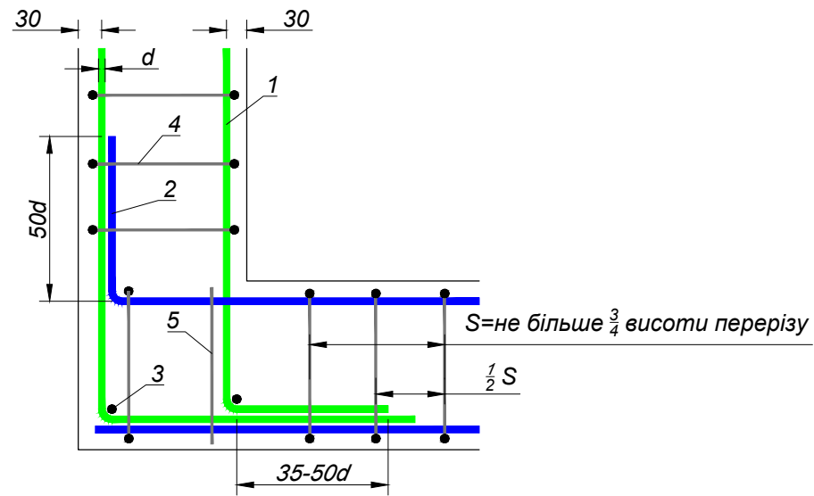
Варіант А. Армуння кута з напуском
