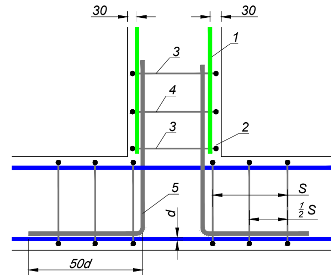
Варіант Ж. Армування примикання Г-подібним хомутом
